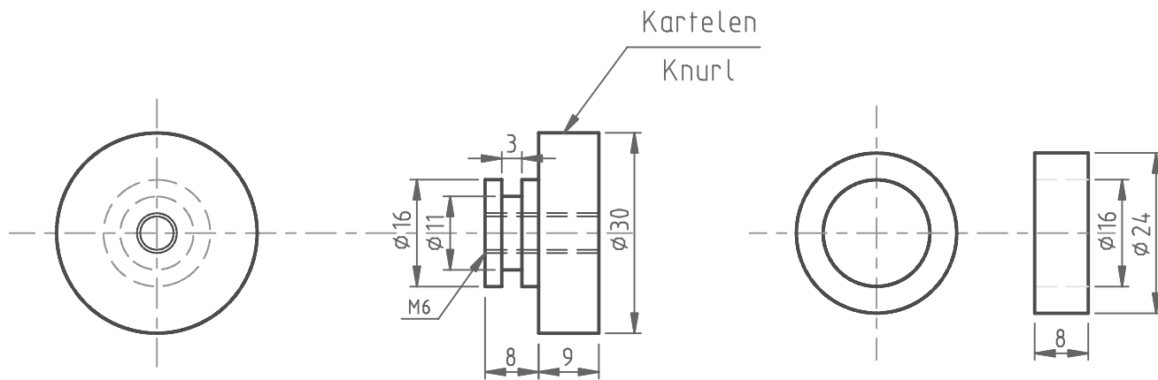
Handwiel Handwheel
