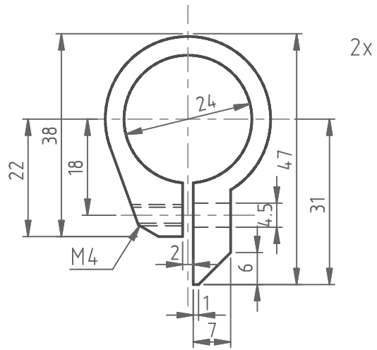
Aanslag - Stopper
