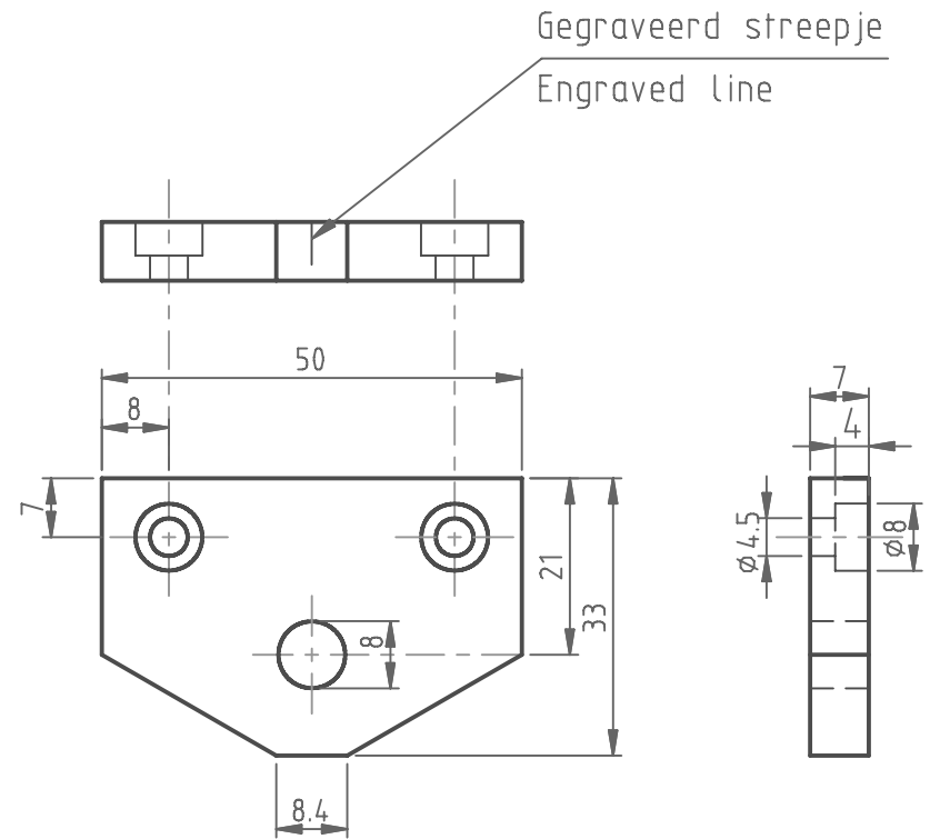
Houder Bracket
